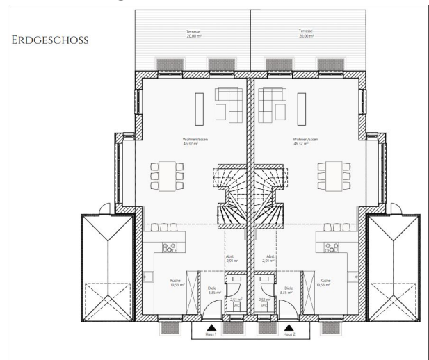
Grundriss Erdgeschoss
