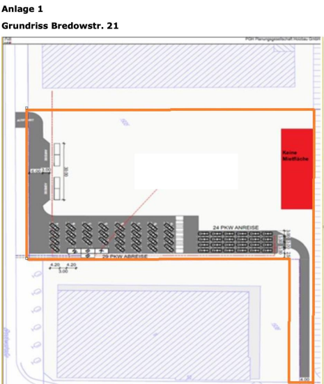
Grundriss Bredowstraße 21
